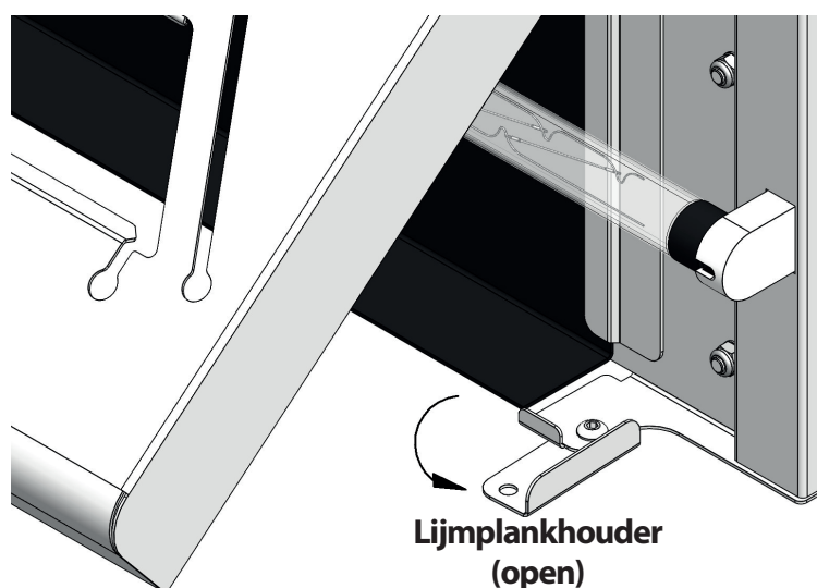
Figuur 2 - Lijmplankhouders
