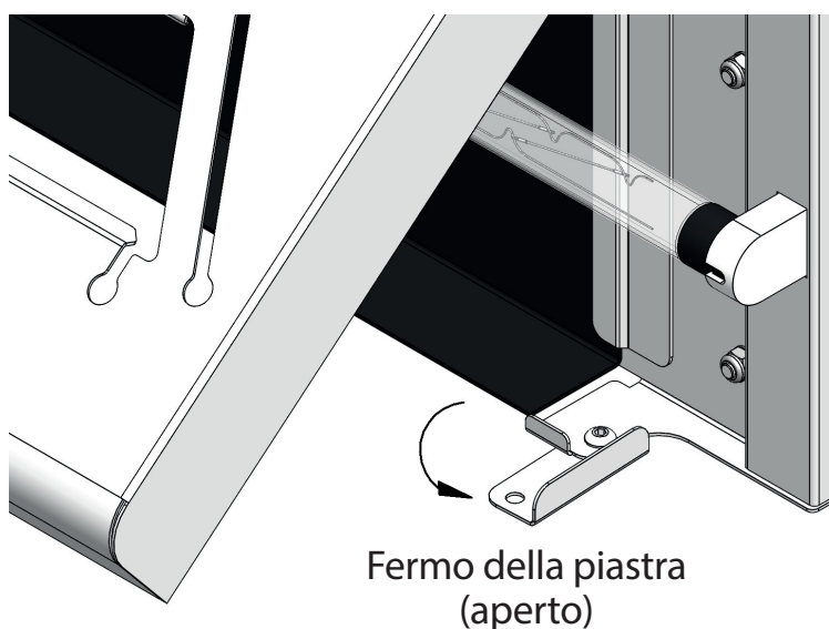
Figura 2 - Fermi della piastra
